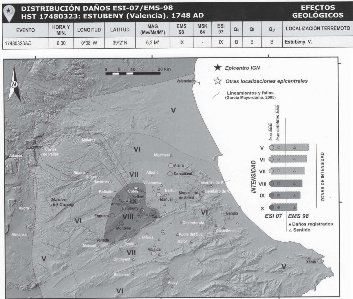
FIGURA 1. DISTRIBUCION DAÑOS.
